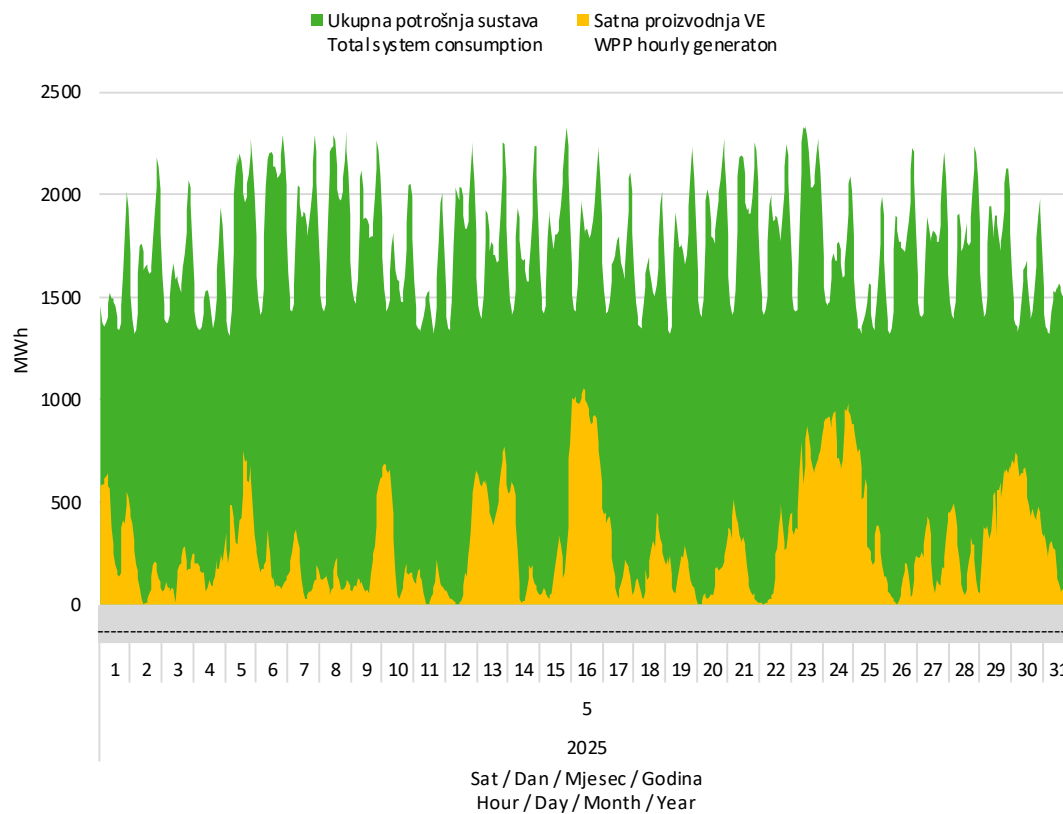
Slika 7 Usporedba satnog dijagrama opterećenja sustava i proizvodnje vjetroelektrana u svibnju 2025. godine
