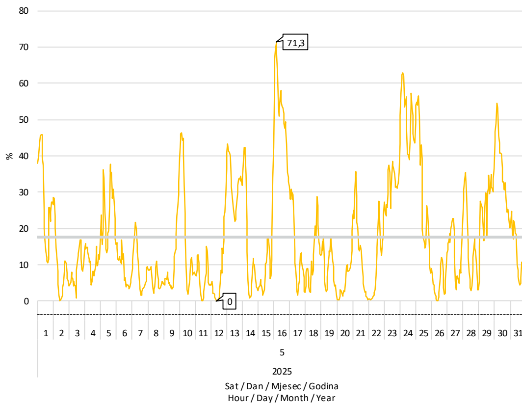
Slika 8 Udio proizvodnje vjetroelektrana u pokrivanju satnog opterećenja elektroenergetskog sustava u svibnju 2025. godine
