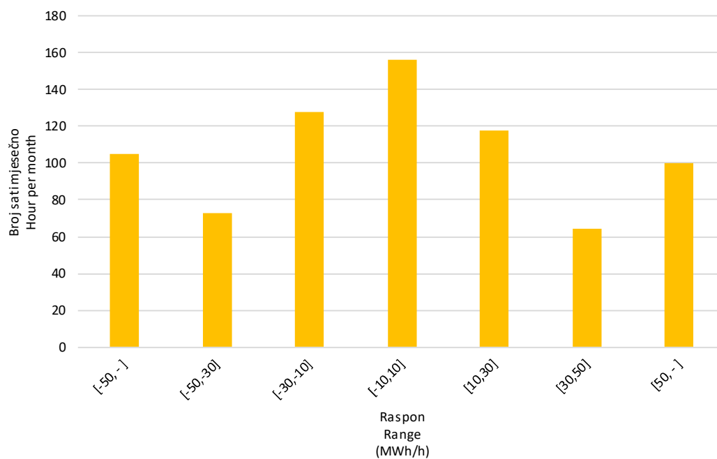
Slika 10 Statistička raspodjela satnih promjena proizvodnje VE u svibnju 2025. godine
