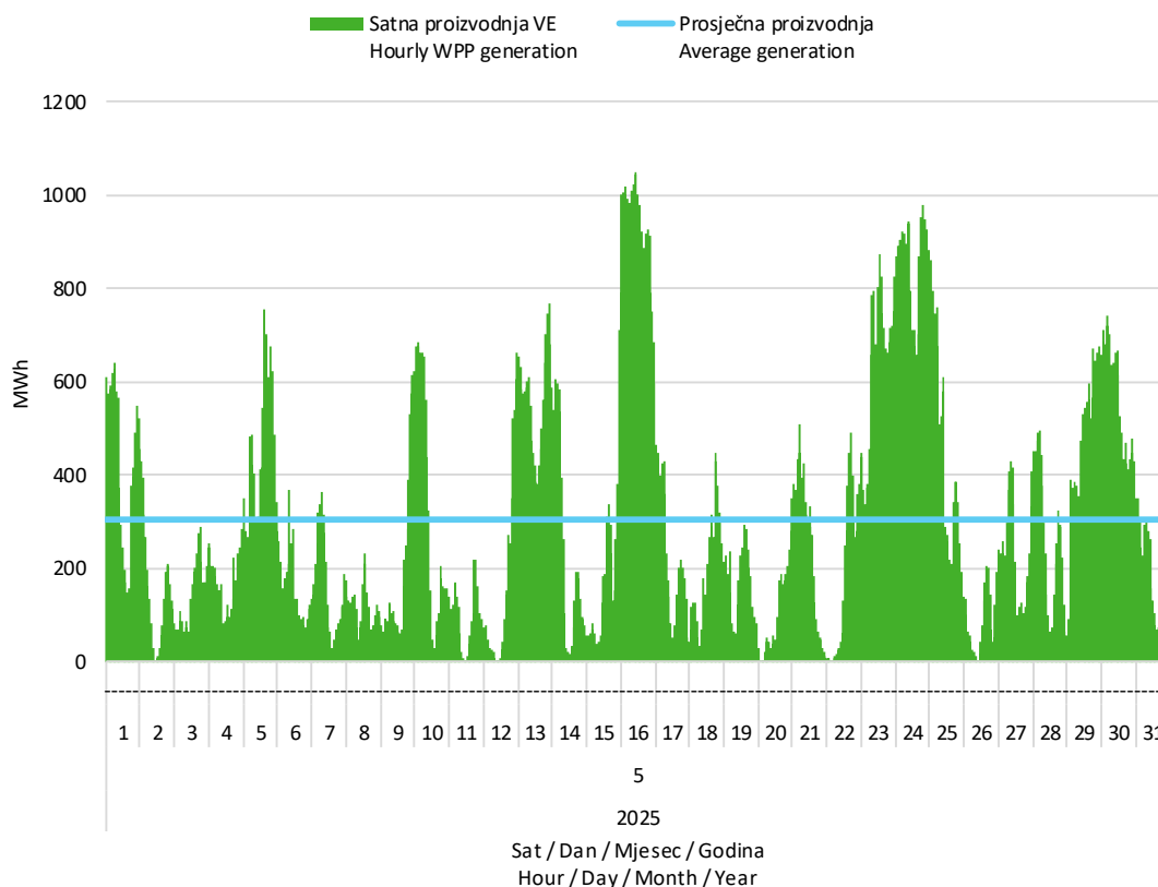
Slika 2 Satna proizvodnja svih vjetroelektrana u svibnju 2025. godine
