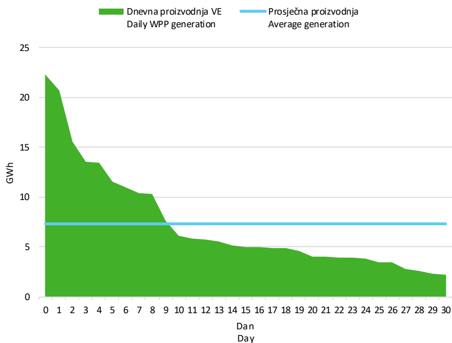
Slika 6 Krivulja trajanja dnevne proizvodnje vjetroelektrana u svibnju 2025. godine
