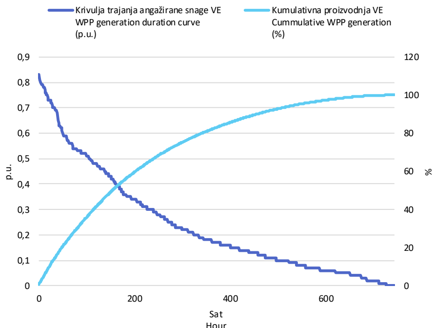
Slika 3 Krivulja trajanja angažirane snage svih VE i kumulativna proizvodnja VE u svibnju 2025. godine u jediničnim vrijednostima
